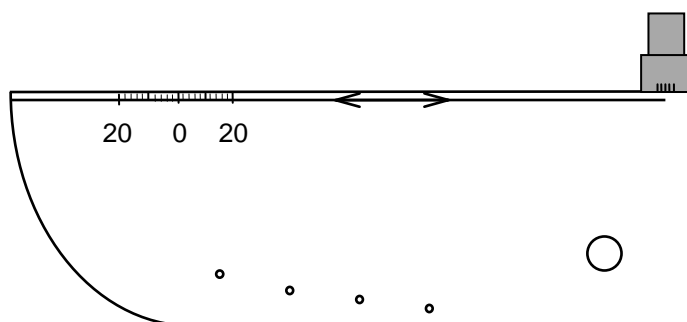
положение ПЭП на образце СО-3Р
