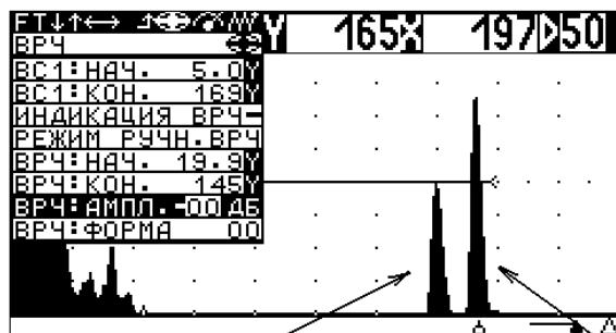
Сигнал от отверстия Сигнал от донной поверхности образца
