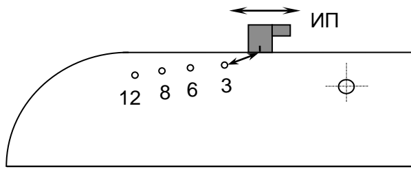
положение ПЭП на стандартном образце СО-3Р
