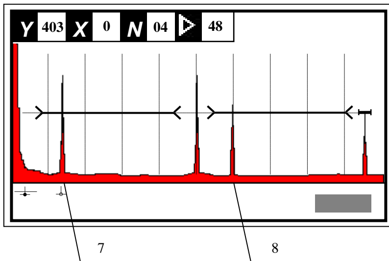
дефект вблизи ПЭП (со стороны излучения)
