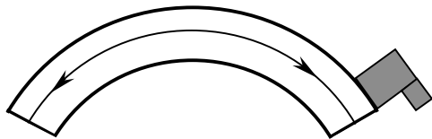
положение ПЭП на СОП для контроля внутренних колец
