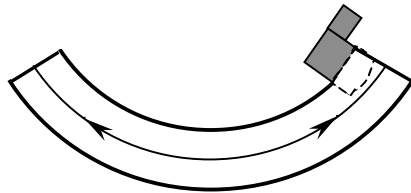
положение ПЭП на СОП для контроля наружных колец
